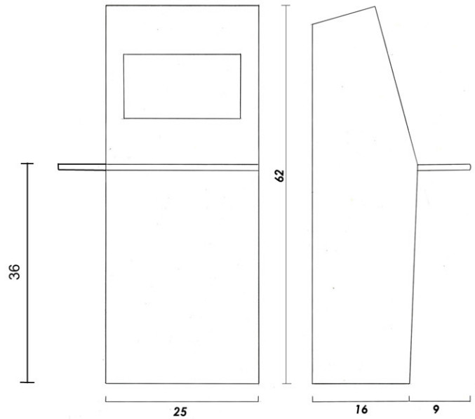
Slimline/Ultraline dimensions
